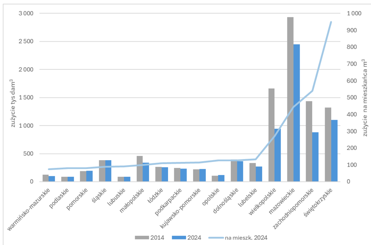
Wykres 101. Zużycie wody na potrzeby gospodarki narodowej
