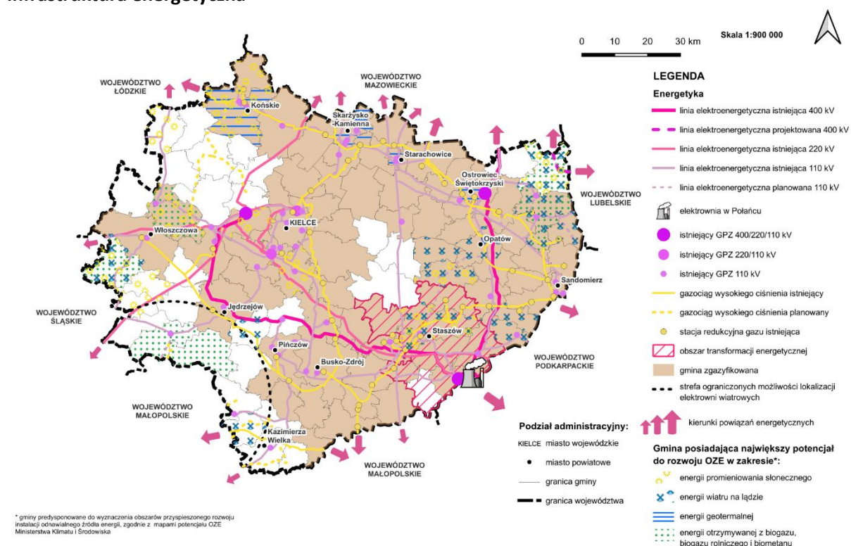
Mapa 4. Model struktury funkcjonalno-przestrzennej województwa świętokrzyskiego – infrastruktura energetyczna
